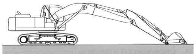
Positie hydraulische-oliepeilcontrole
