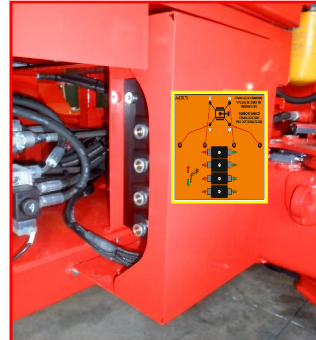
Afbeelding 36: bedieningspaneel stempelpoten.
